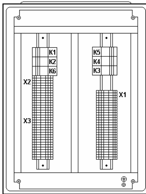
монтажная панель
