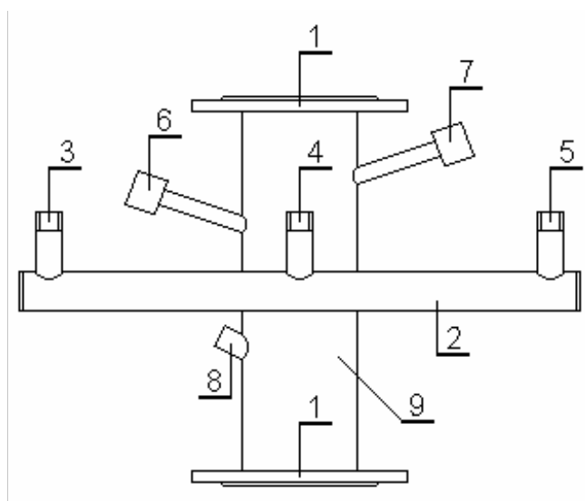
Рис. 4. Вертикальный отвод для установки группы безопасности.
