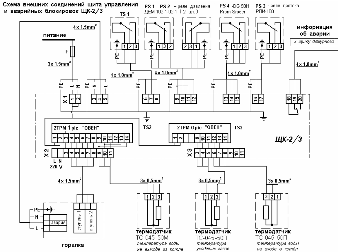
Рис. 3. Схема внешних соединений щита.
