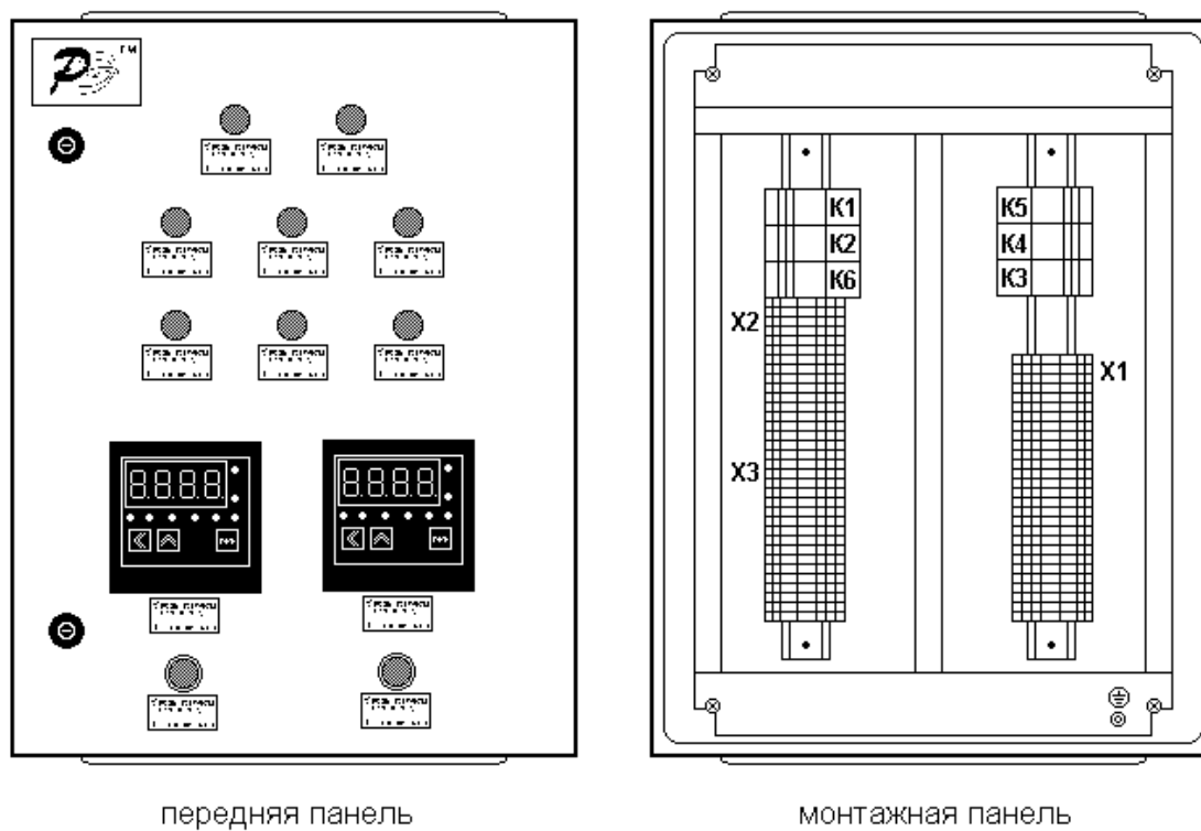
Рис. 1. Щит управления и аварийных блокировок.
