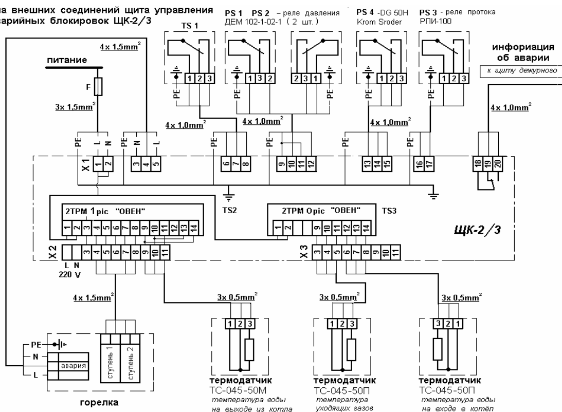
Рис. 3. Схема внешних соединений щита.
