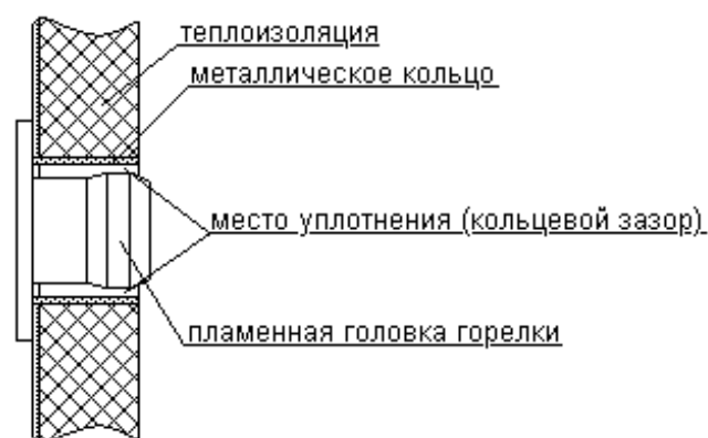
Рис. 5. Фрагмент фронтальной крышки котла (уплотнение зазора между крышкой и пламенной головкой).
